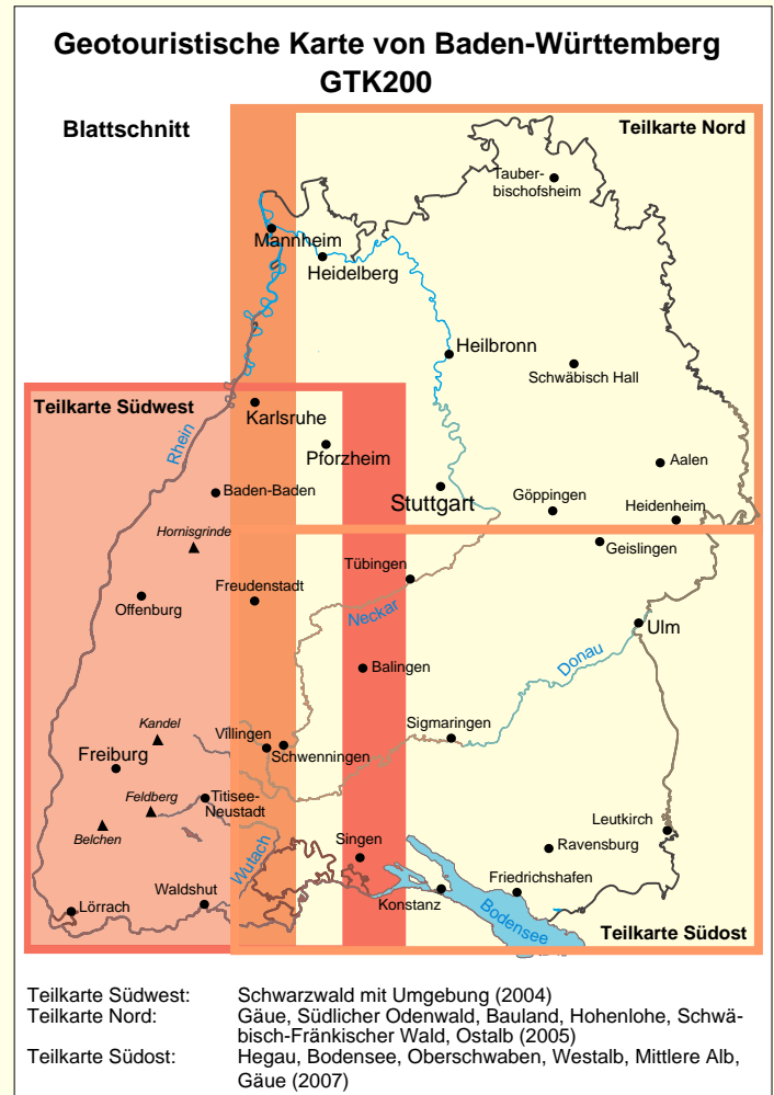
Abb. 1: Landesübersicht mit Blatteinteilung der GTK200
